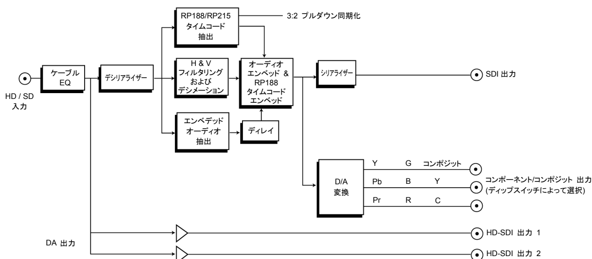
HD10MD3 HD → SDI ダウンコンバーター ブロックダイアグラム
